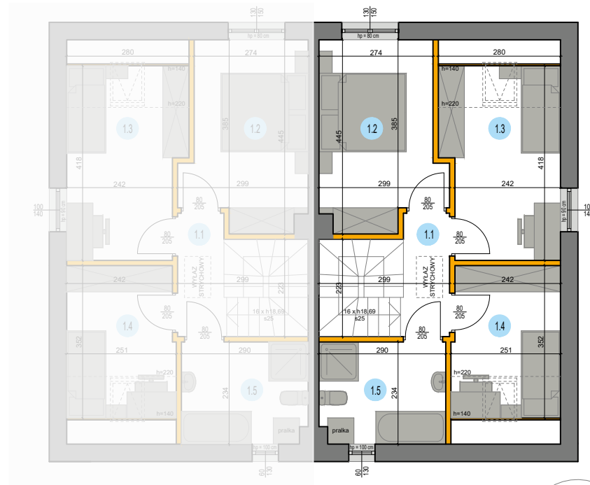
LOKAL 2 - PIĘTRO
