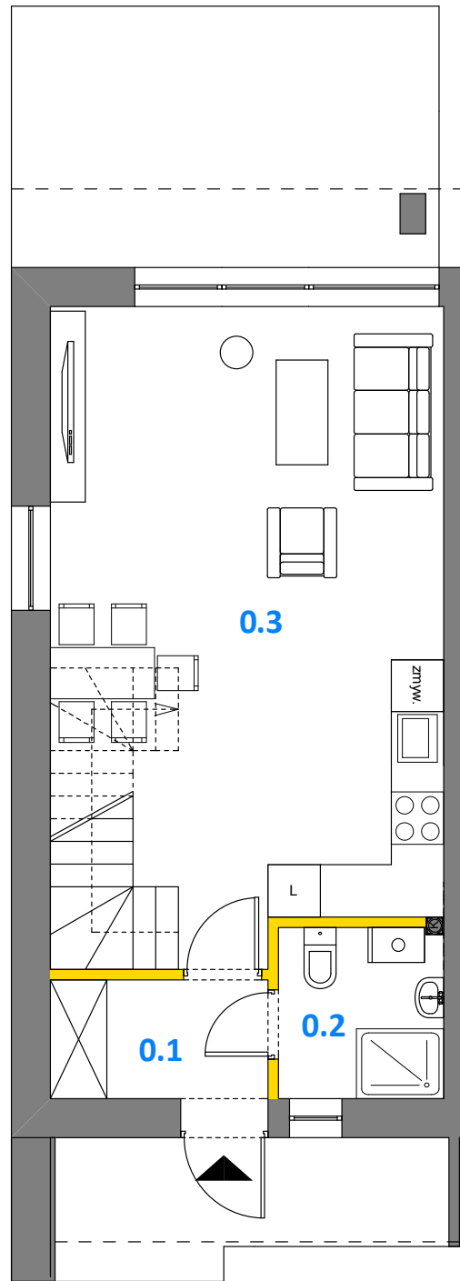
RZUT PARTERU
