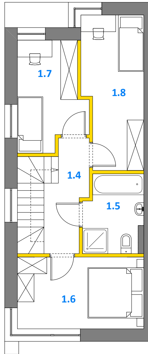
RZUT PIĘTRA
